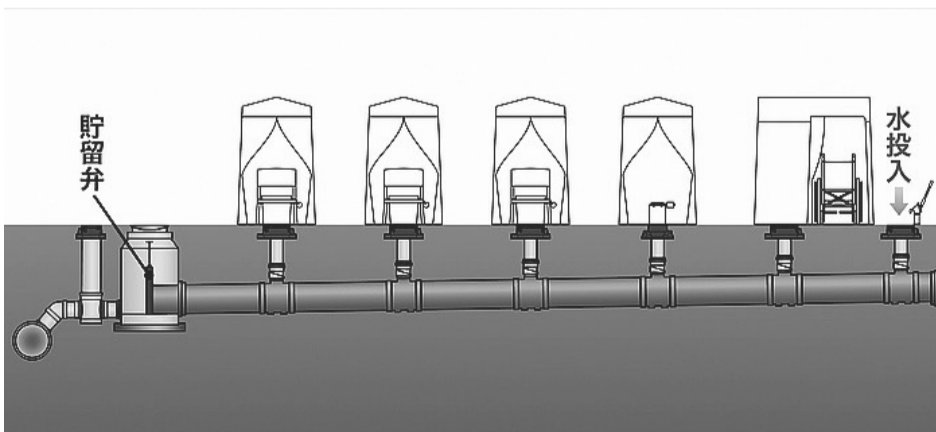
マンホールトイレの仕組み
